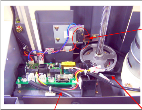
26 : 【EMAMS0305 マイクロスイッチ (AM50054C5)】 (上限・下限・安全SW部に使用)
