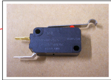
26 : 【EMAMS0305 マイクロスイッチ (AM50054C5)】 (上限・下限・安全SW部に使用)
