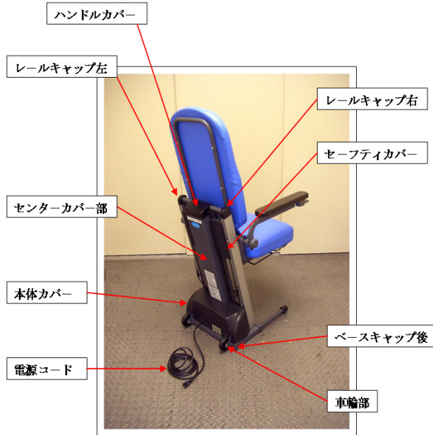
背面各部
