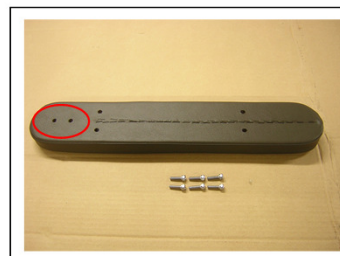
3-1 : 【62651302 アームレストR 新エコライト用 (組付ネジ付) 組付ネジセット (M6×20) 6本 裏面の取付箇所 (赤丸枠内を含め6箇所)
