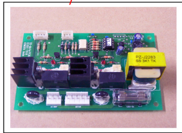
25 : 【61681701 ACモーター制御基板】
