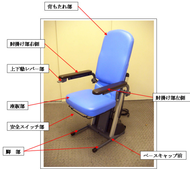
正面側各部
